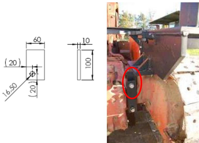
Figura 5. Elemento A2
