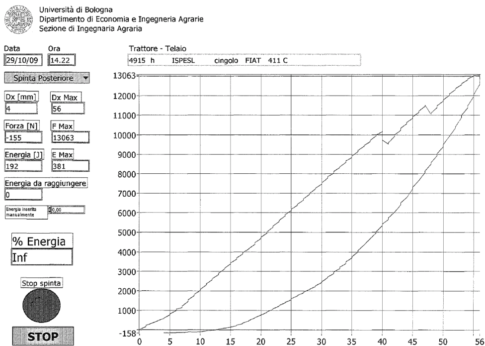
Figura 20. Spinta longitudinale posteriore
