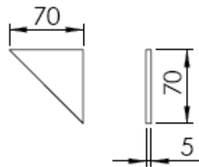
Figura 15. Elemento T3.
