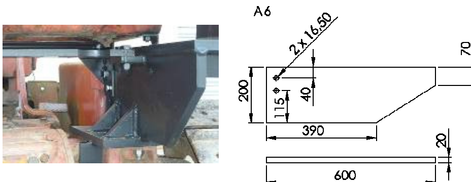
Figura 9. Elemento A6.
