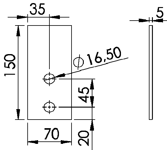
Figura 14. Elemento T2.
