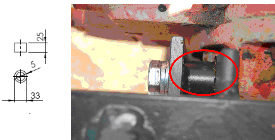
Figura 6. Elemento A3
