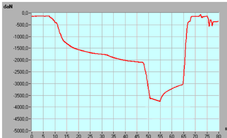
Figura 15. Primo schiacciamento
