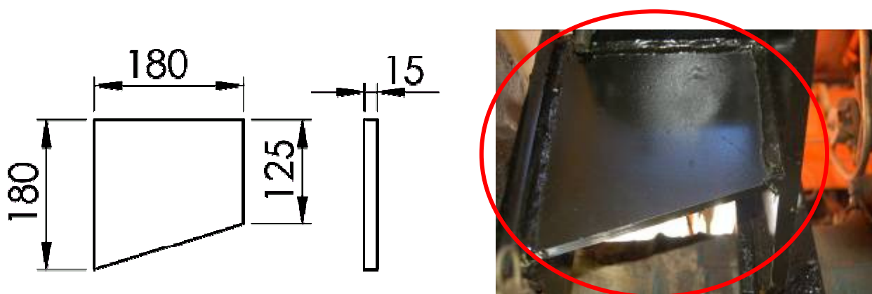
Figura 7. Elemento A5
