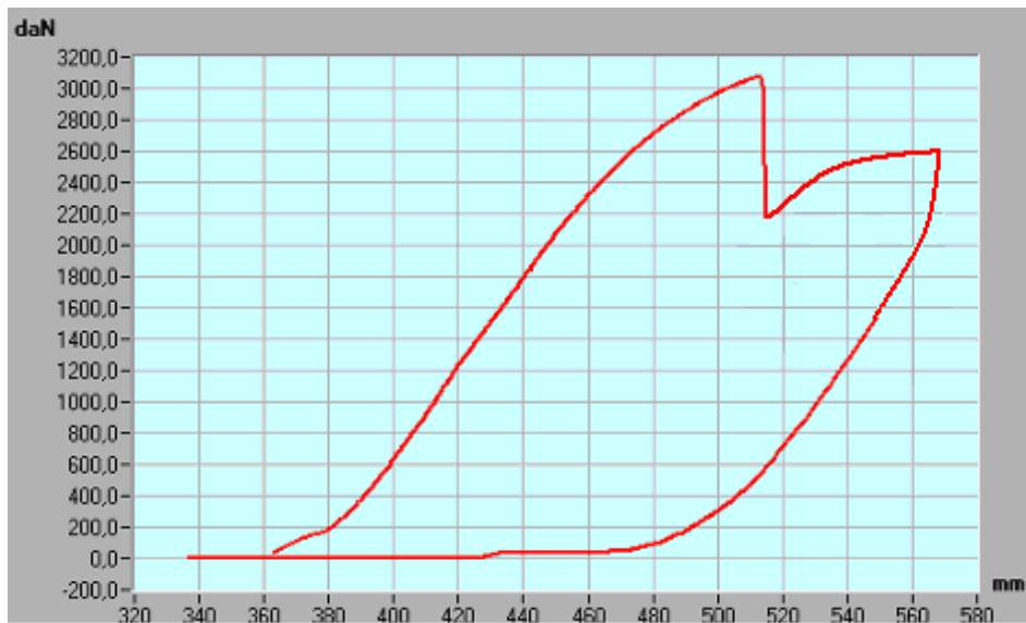
Figura 16. Spinta laterale lato sinistro
