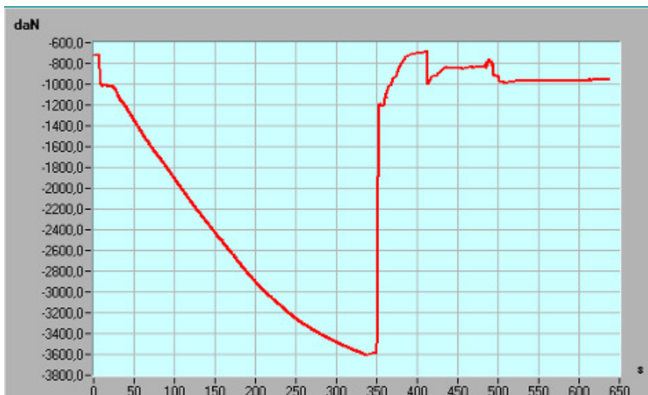
Figura 17. Secondo schiacciamento
