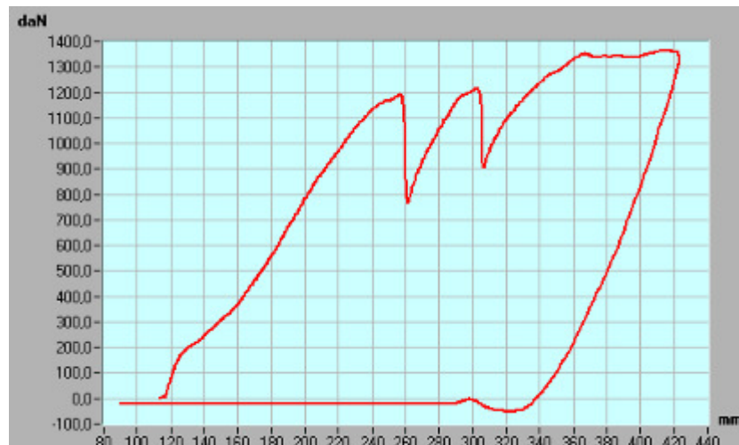
Figura 14. Spinta posteriore lato destro
